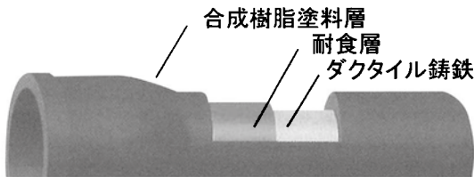
外面耐食仕様C-Protect(イメージ図)
