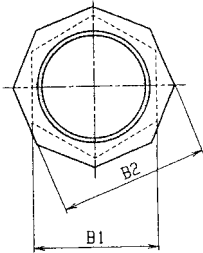
袋ナット
