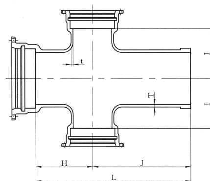
呼び径500～900
