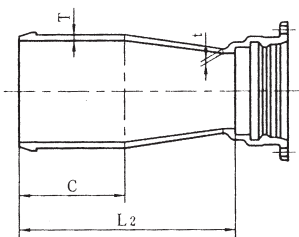
呼び径 300 ～ 450
