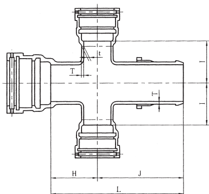
呼び径75～250
