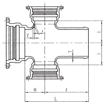
呼び径300～450
