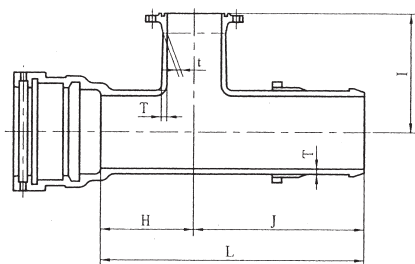
呼び径75～250
