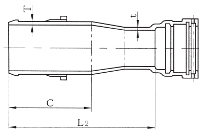
呼び径 100 ～ 250
