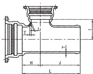
呼び径300～450
