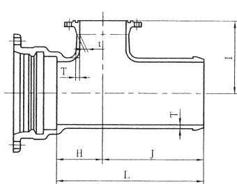
呼び径300～450
