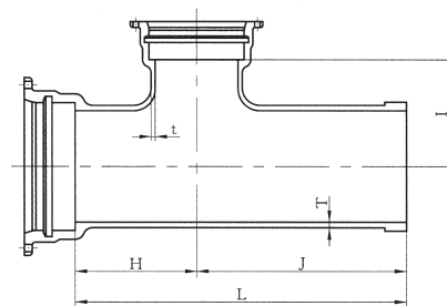
呼び径500～1000
