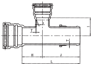
呼び径75～250
