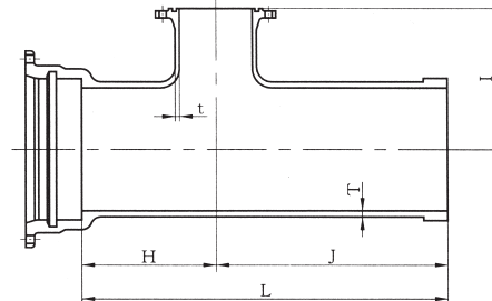
呼び径500～1000
