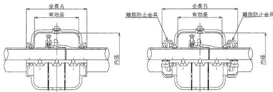
ø200～ø400 (三つ割) CJC／1 (標準仕様) CJC／1-S (離脱防止金具付き)
