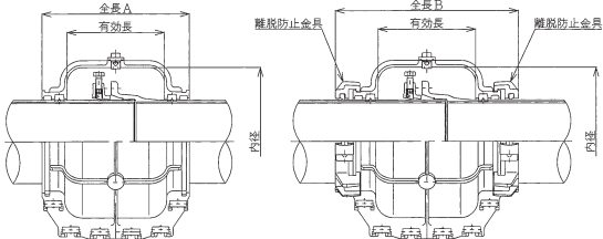
ø200～ø400 (三つ割) CJC／1 (標準仕様) CJC／1-S (離脱防止金具付き)
