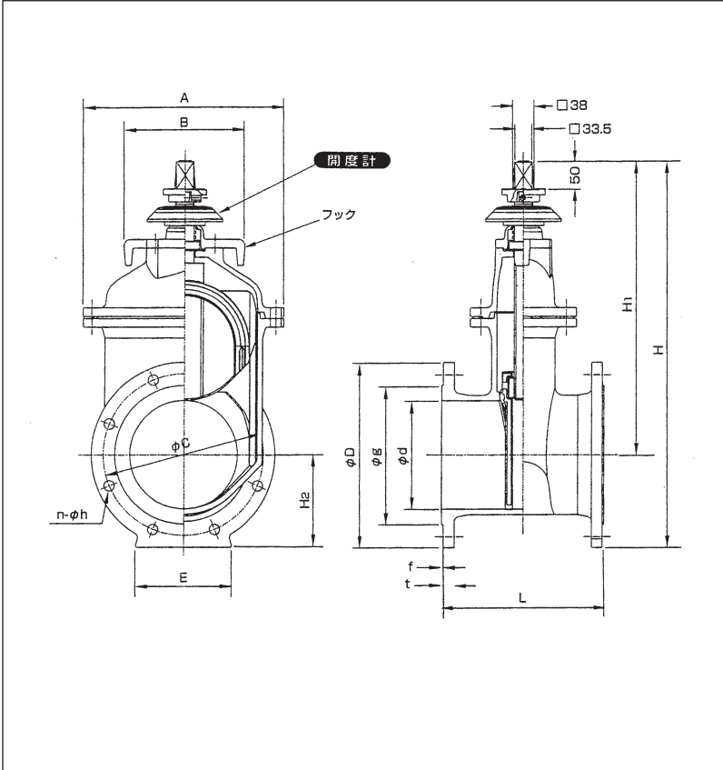
各部寸法 単位: mm
