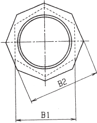
袋ナット
