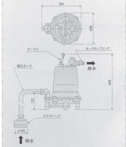
■外形寸法図 (単位:mm)
