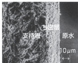
セラミック膜の断面（電子顕微鏡）
