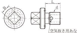
空気抜き用ボルト及び水抜き用ボルト (SUS304)
