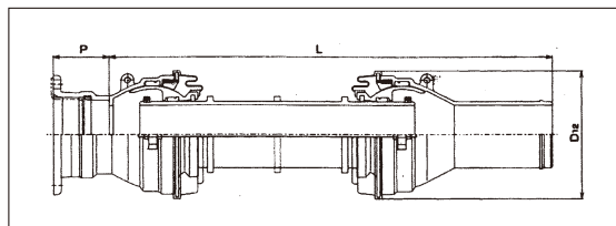
●EB-SGSG 鑄鉄管GX形挿口×鑄鉄管GX形挿口
