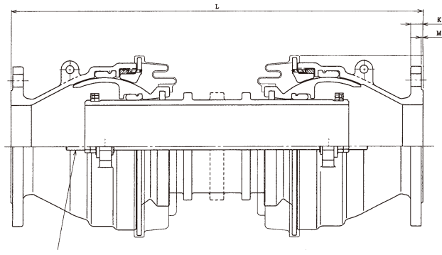
タイロッド
