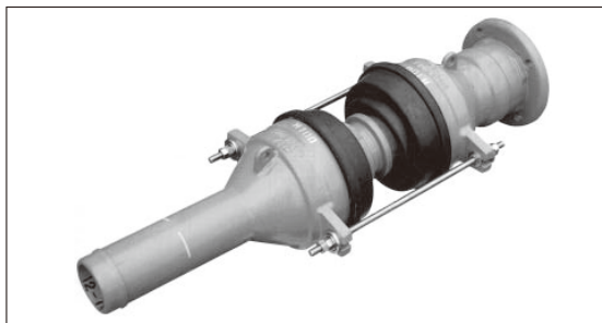
●EB-UGUG 鑄鉄管GX形受口×鑄鉄管GX形受口
