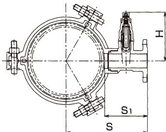
呼び径 250～400×50 寸法図
