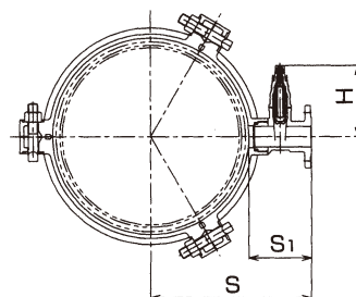
呼び径 450～600×50 寸法図
