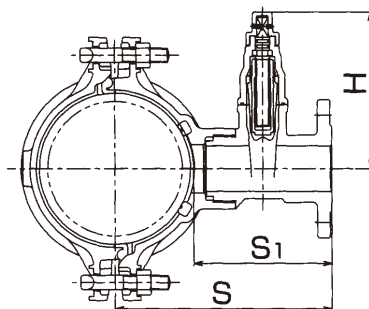
呼び径75～200×50寸法図
