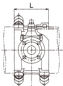
呼び径 250～400×50 寸法図
