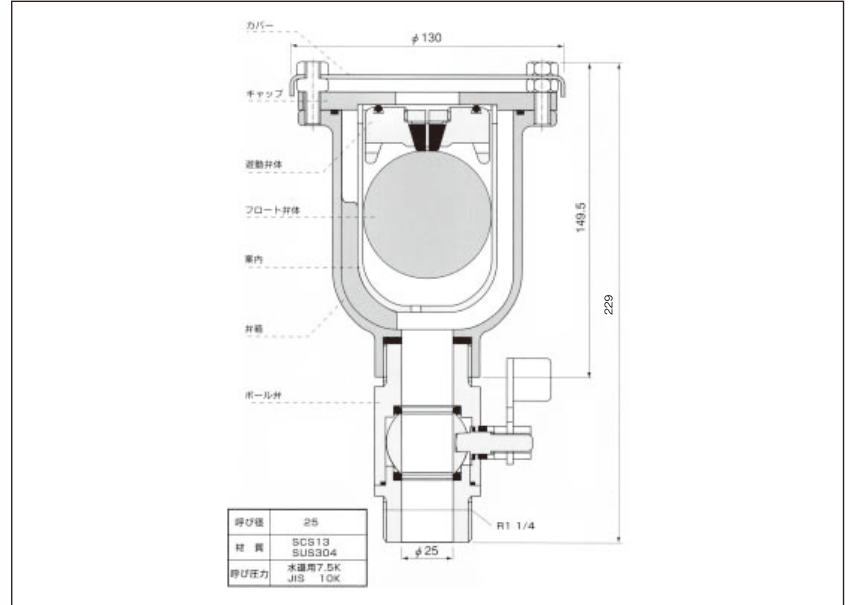
寸法図
