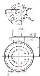
(ステム部詳細図)
