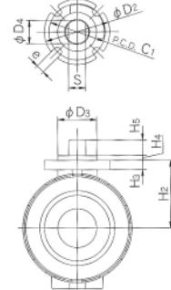
(ステム部詳細図)
