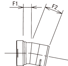
11°エルボ
