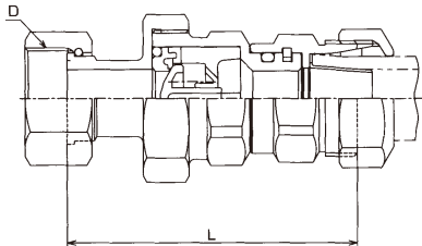
●主要部寸法表
