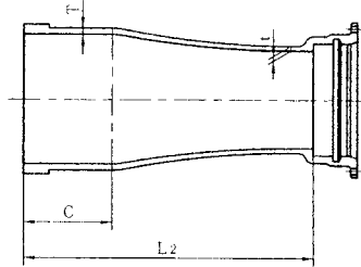
呼び径 500 ~ 1000
