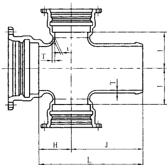
呼び径300~450
