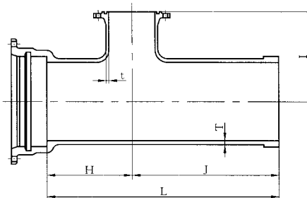
呼び径500~1000
