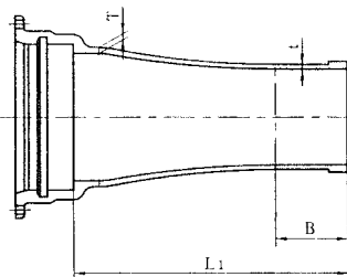
呼び径500~1000
