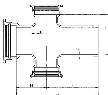
呼び径500~900
