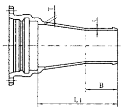
呼び径300~450
