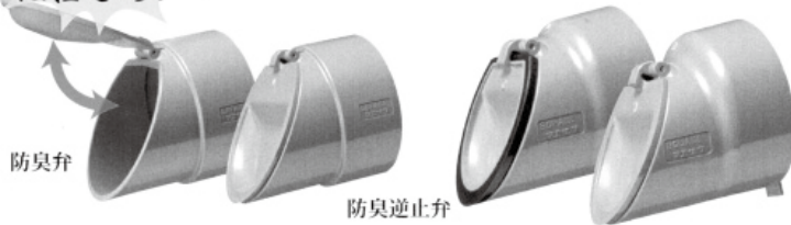
防臭逆止弁
