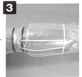
3 管理設位置に地下水が存在する場合は継手部に固定ネットを取り付けます。
