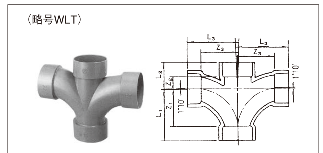
VP系(品番2156)=VP系ストッパー=
