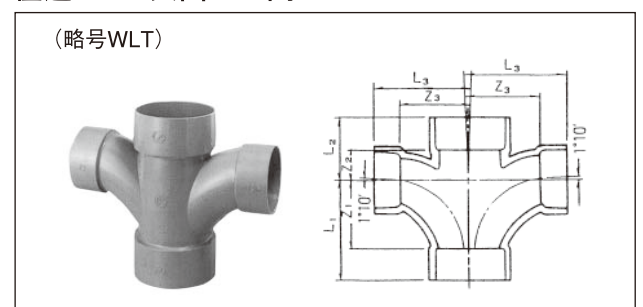
VP系(品番2156)=VP系ストッパー=
