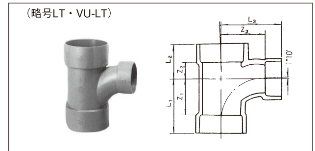
VP系(品番2155)=VP系ストッパー=
