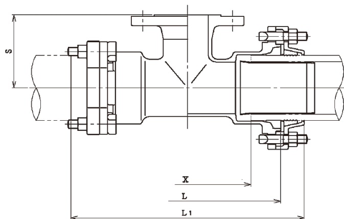
呼び径150・200の形状
