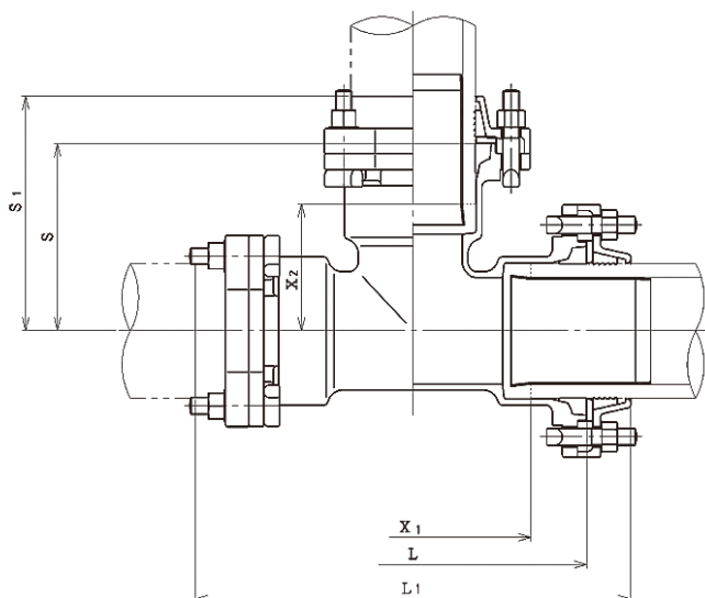
呼び径150・200の形状
