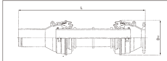
●EB-FSG 鑄鉄管フランジ形×鑄鉄管GX形挿口
