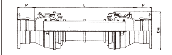
●EB-FUG 鑄鉄管フランジ形×鑄鉄管GX形受口
