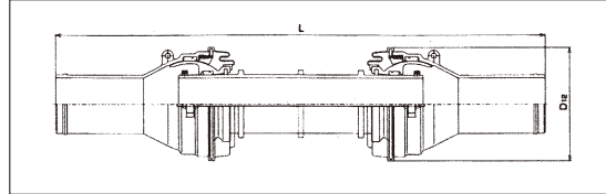
●EB-FSG 鑄鉄管フランジ形×鑄鉄管GX形挿口
