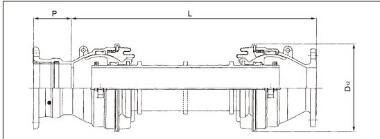
●EB-FUG 鑄鉄管フランジ形×鑄鉄管GX形受口
