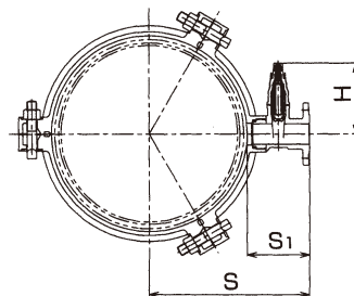
呼び径 450～600×50 寸法図
