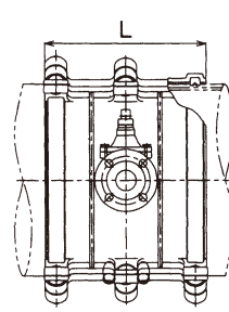
呼び径 450～600×50 寸法図
