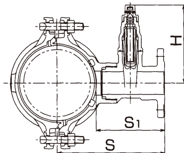
呼び径75～200×50寸法図
