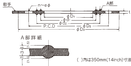
アサヒAVパッキン寸法図 (全面用)
