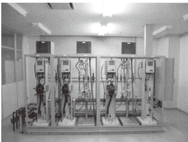
計装機器設備
