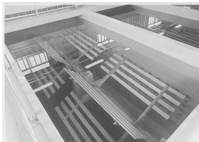
フロキュレーター
