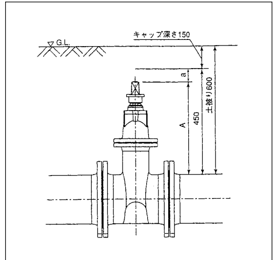
■浅層埋設の対応 (土被り600mmの場合)
