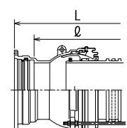
300以上の形状 受口 NS形 (UN)
