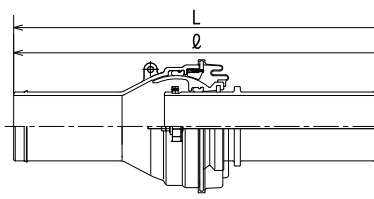
挿口 NS形種管 (SNE)
