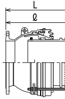
フランジ (F)
