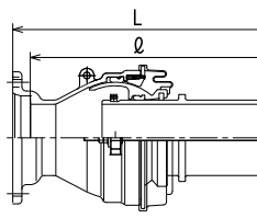
受口 NS形種管 (UNE)
