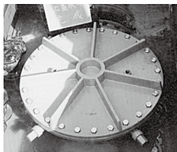
インサープラグⅠP
