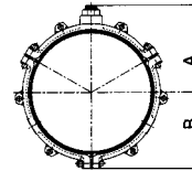
呼び径450~700mm(鋳鉄管用・水抜きボルト付)
