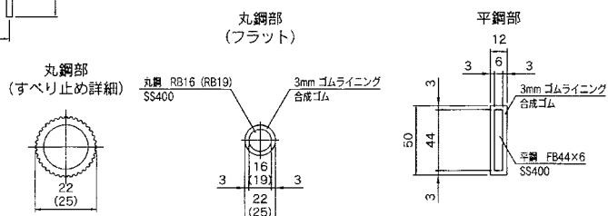
ゴムライニング部詳細図
