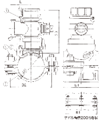
サドル機構50・75の形状 サドル機構150の形状 サドル機構200の形状
