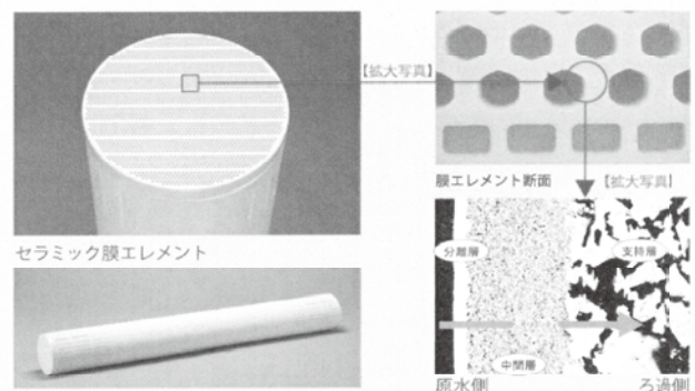
セラミック膜の構造
